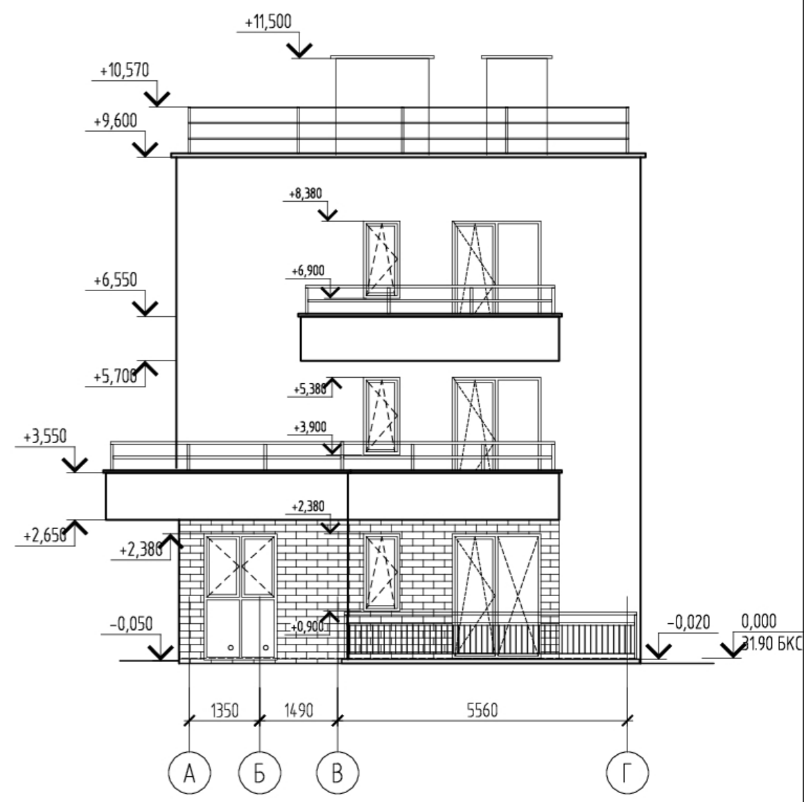
Фасад в осях А-Г.
