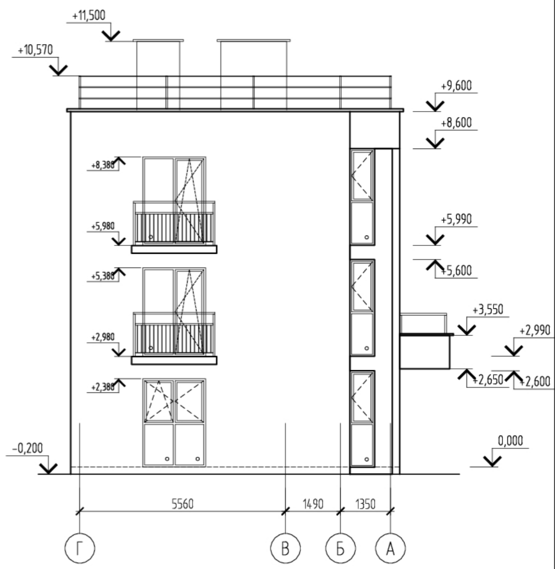
Фасад в осях Г-А.
