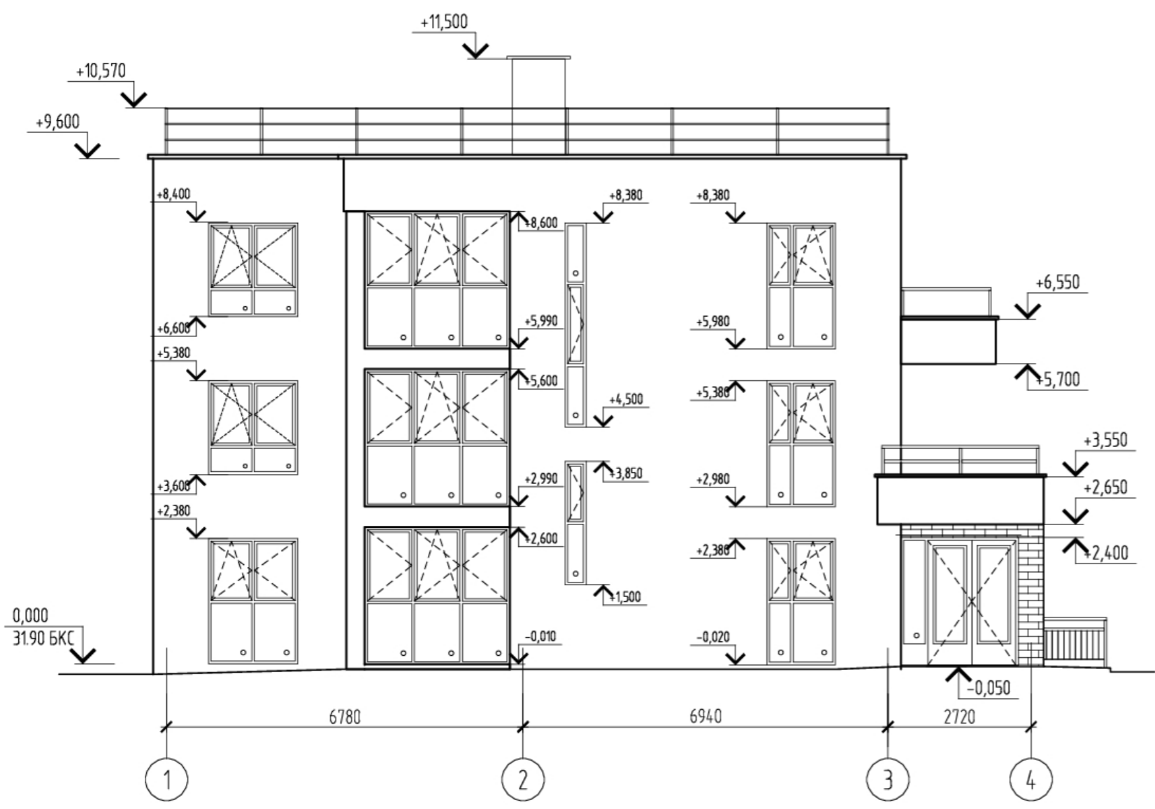
Фасад в осях 1-4.
